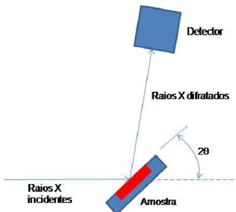
Figura 2. Desenho esquemático da detecção de XRD.
