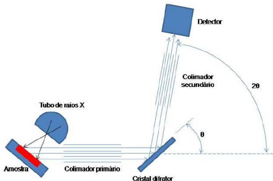
Figura 1. Desenho esquemático da detecção de XRF.
