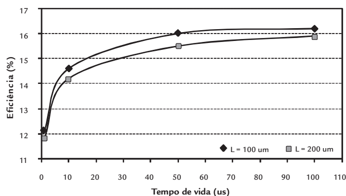
Figura 2 Eficiência das células solares processadas em Si-mc, em função do tempo de vida dos minoritários para L = 100 \mu m e L = 200 \mu m.
