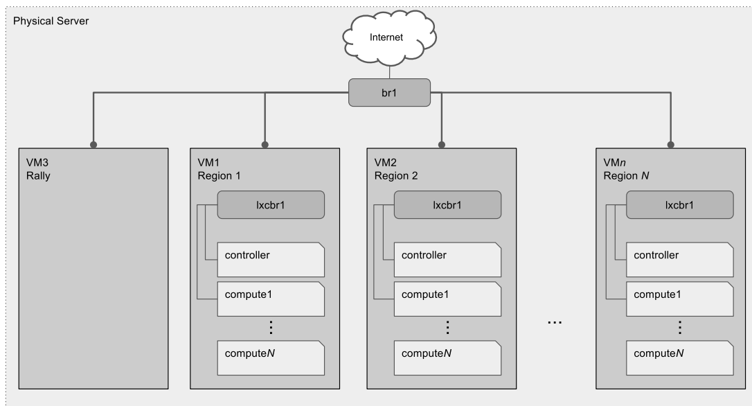
Figura 3. Topologia física do experimento
