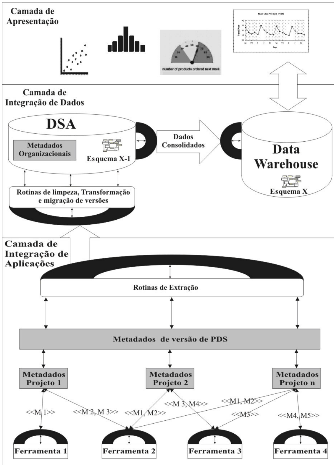
Fig. 6. Arquitetura de Data Warehousing para PDS em evolução
