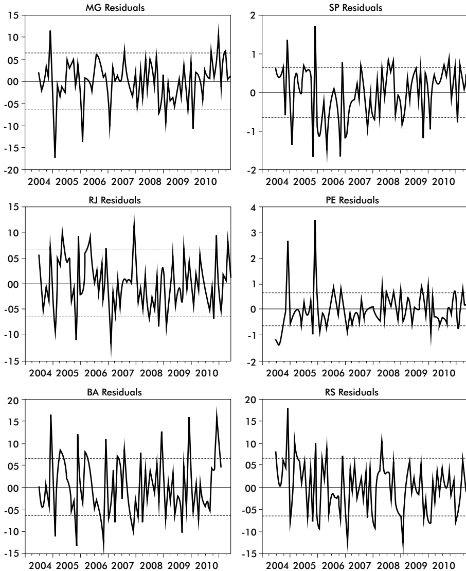
Figura 1 – Gráfico dos resíduos da estimação em painel
