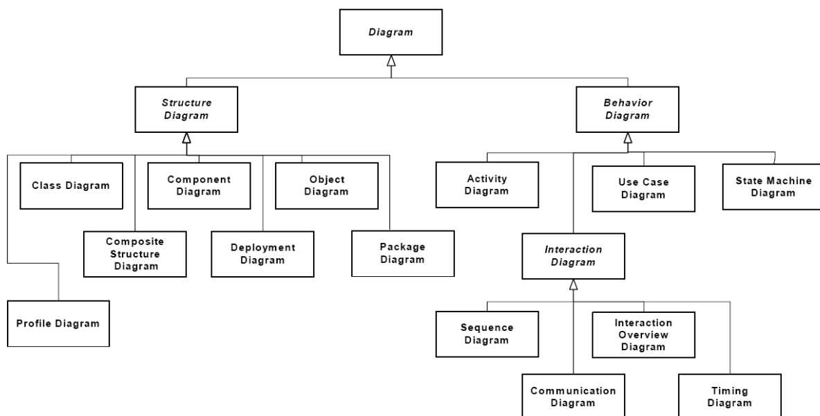
Figura 3 – Categorização dos diagramas UML
