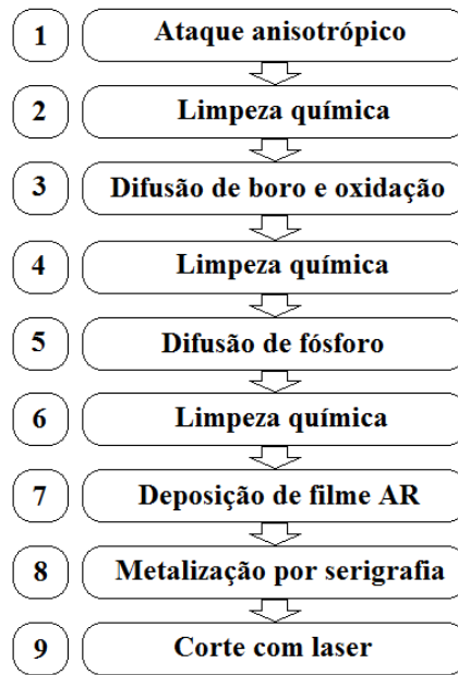
Figura 3 - Etapas do processo de fabricação de células solares do tipo n^+np^+ .
