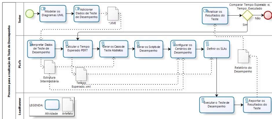
Figura 1. Processo da abordagem de teste de desempenho baseado em modelos
