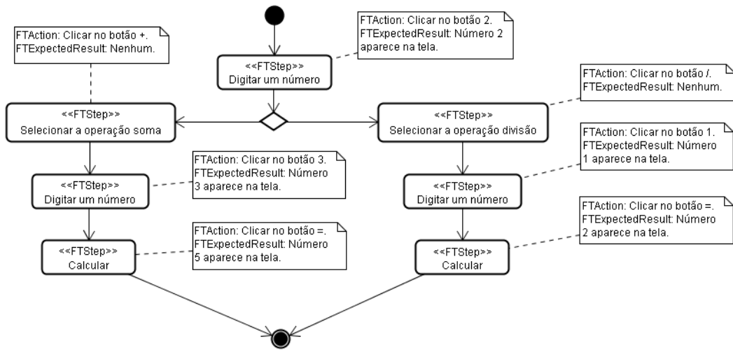
Figura 5. Diagrama de atividades após a composição.
