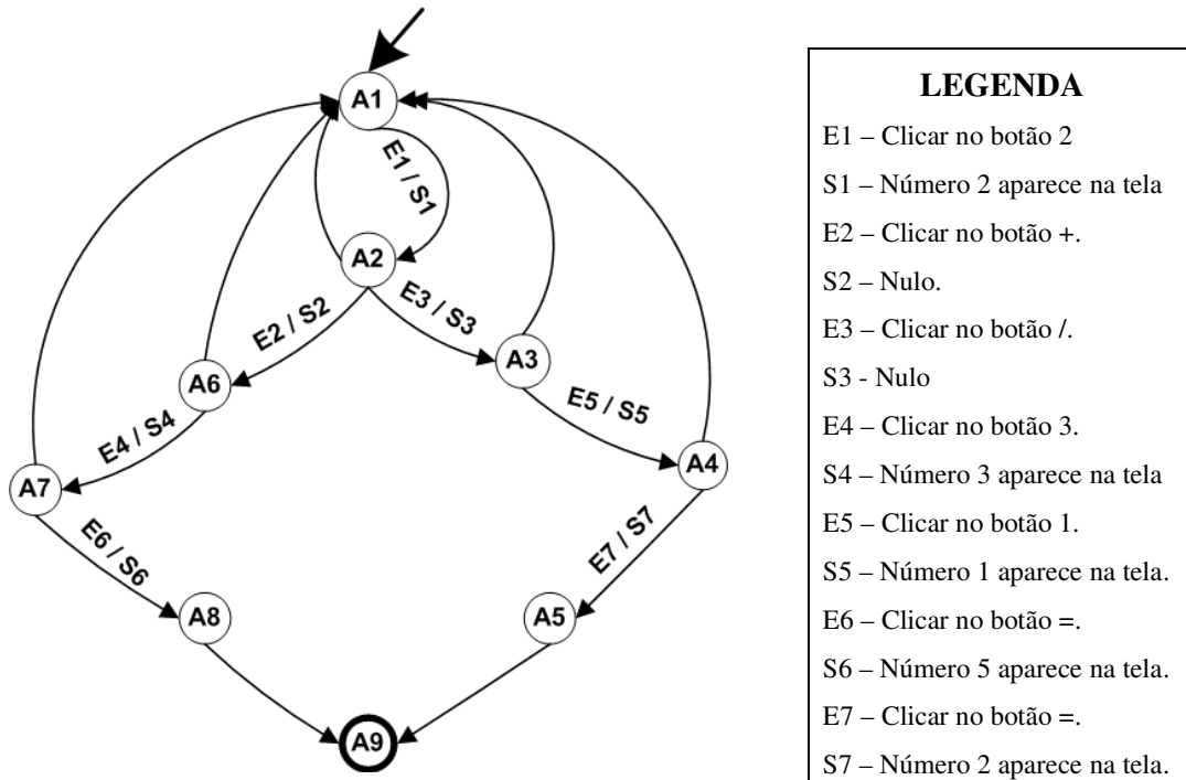
Figura 6. Máquina de estados finitos equivalente.
