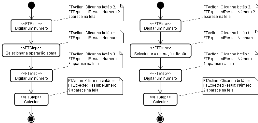
Figura 4. Diagramas de atividades referentes aos casos de uso Somar e Dividir .
