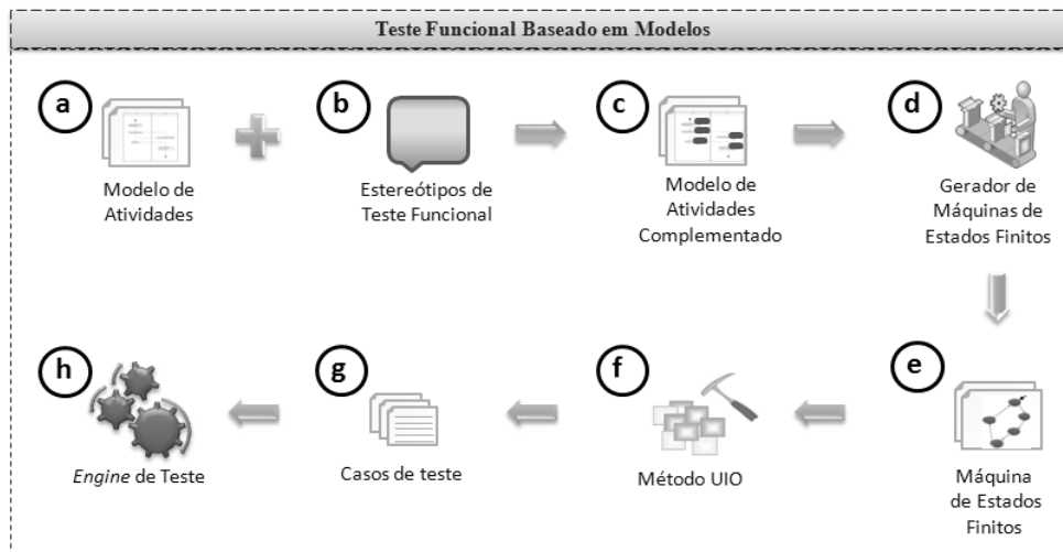
Figura 1. Um overview da abordagem proposta.
