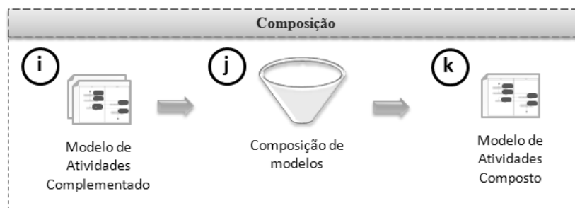
Figura 2. Processo de composição dos diagramas de atividades.
