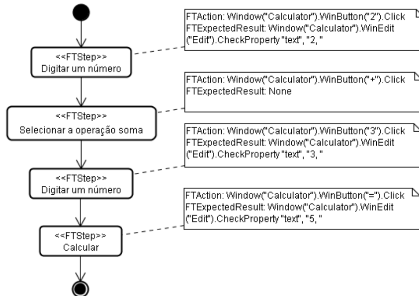
Figura 7. Diagrama de atividades referente aos casos de uso Somar , dotado de comandos da ferramenta Quick Test Professional.
